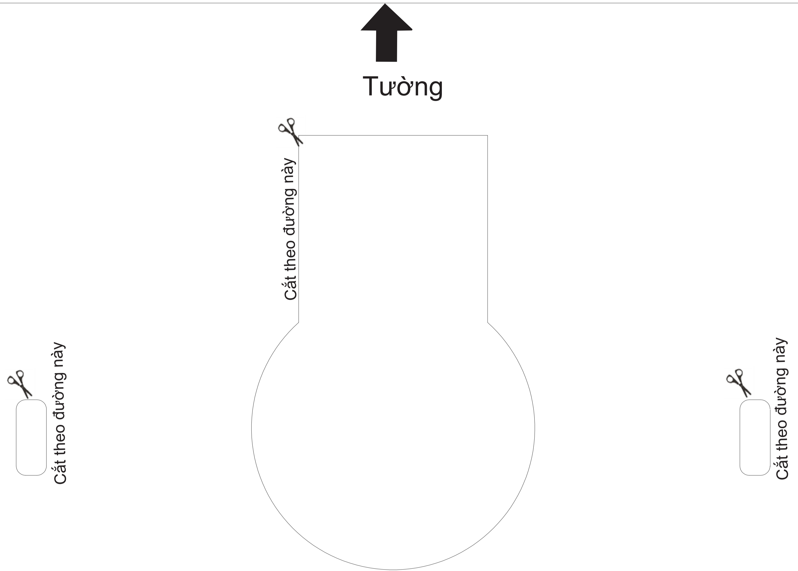
Hình 1: Bản vẽ tỷ lệ 1:1 sử dụng để cắt lỗ lắp đặt chậu lên bàn
